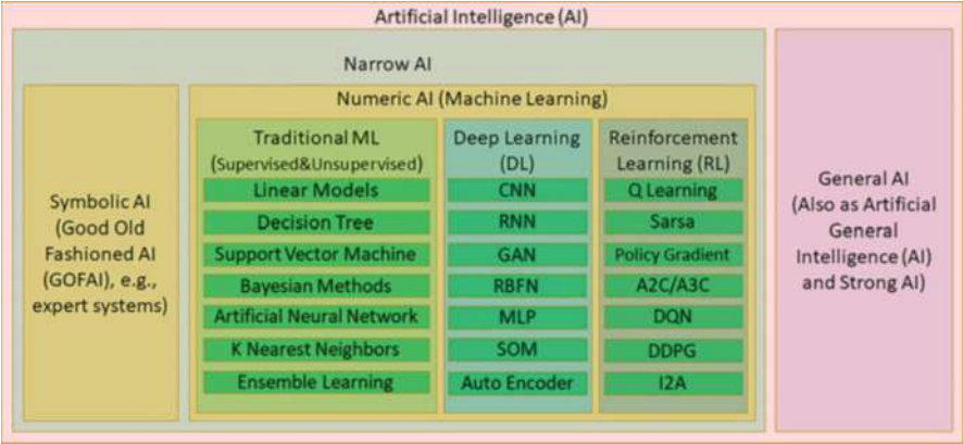
Fig. 1.1 Subareas in AI
